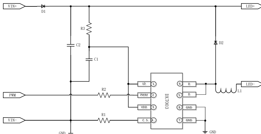
图 4.1 DX7003 应用电路
