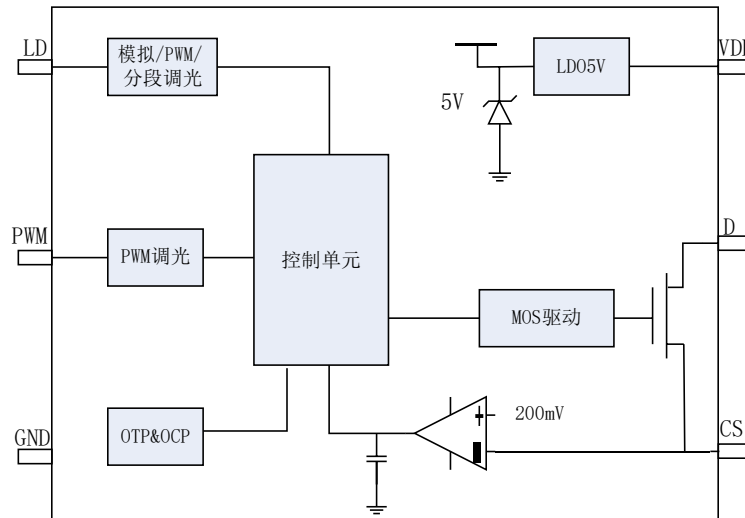
图 7.1 结构框图
