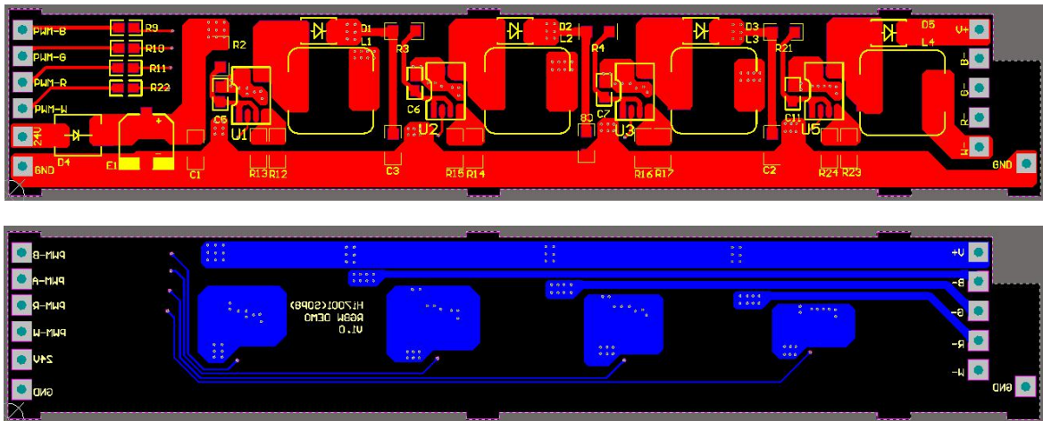
图 11.2 四路 RGBW 共阳连接电路布局布线图
