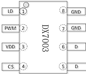
图 5.1 DX7003 管脚图
