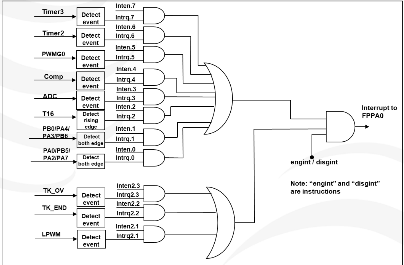
图 15: 中断硬件框图
