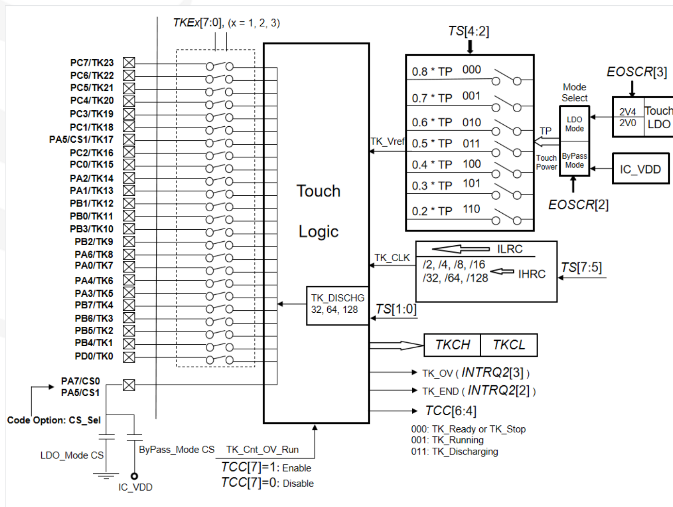
图 41: 触摸检测电路的功能方框图
