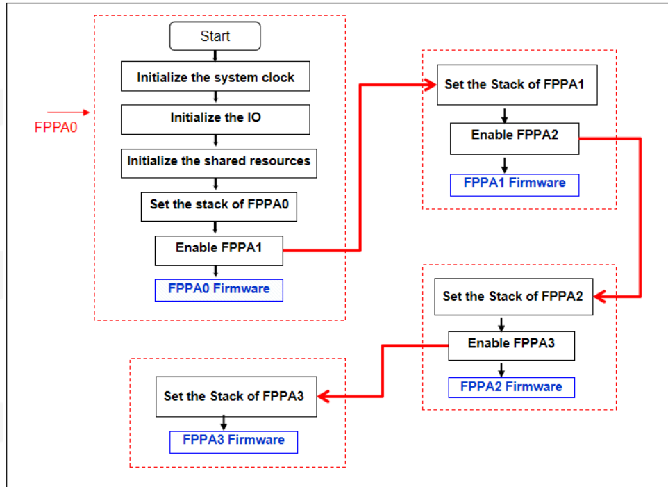
图 11: 开机流程
