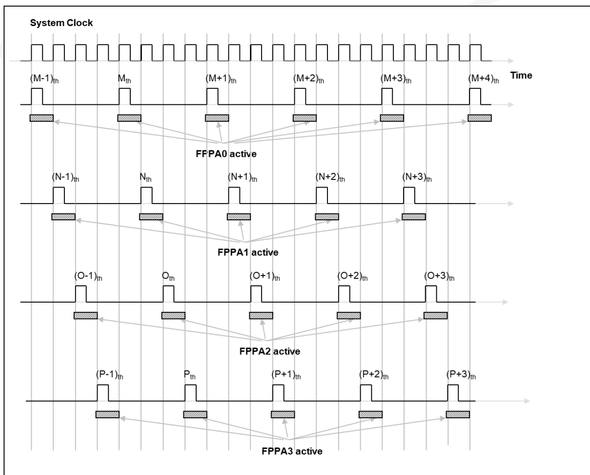
图 2：4-FPPA 单元架构以及基本时序
