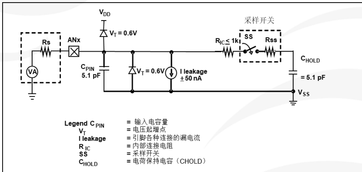
图 39：模拟输入模型
