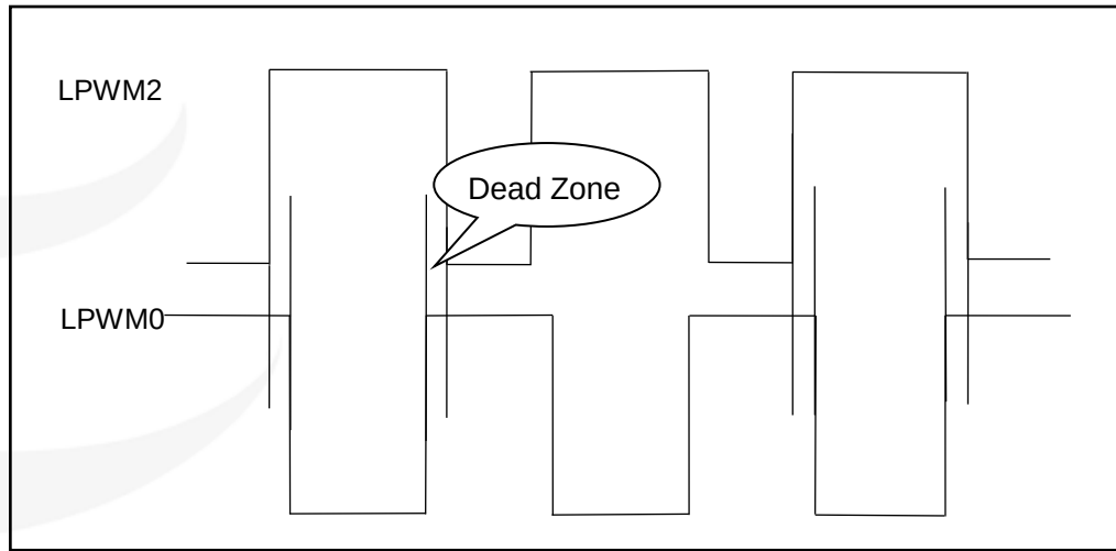
图 27：两路互补 LPWM 波形
