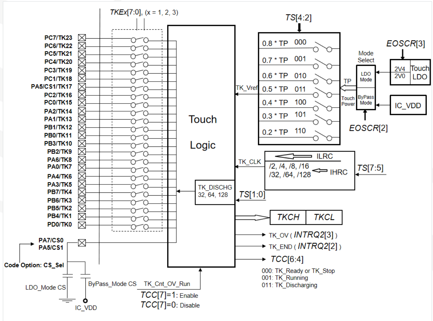
图 41：触摸检测电路的功能方框图
