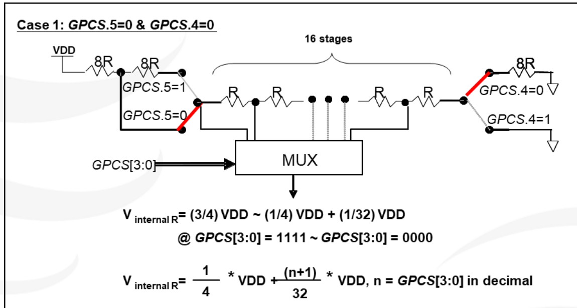
图 31: V_{\text{internal R}} 硬件接法 ( \text{GPCS}.5=0 & \text{GPCS}.4=0 )
