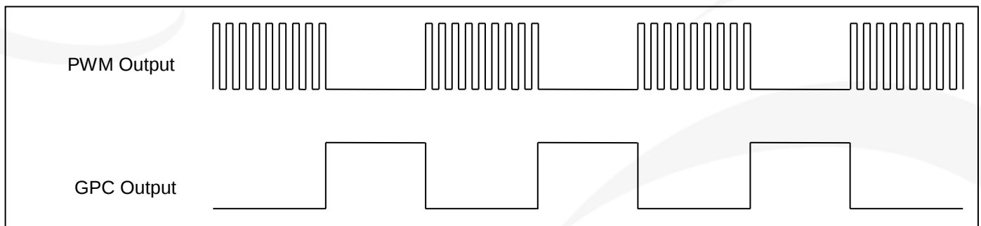
图 30: 比较器结果控制 PWM 输出
