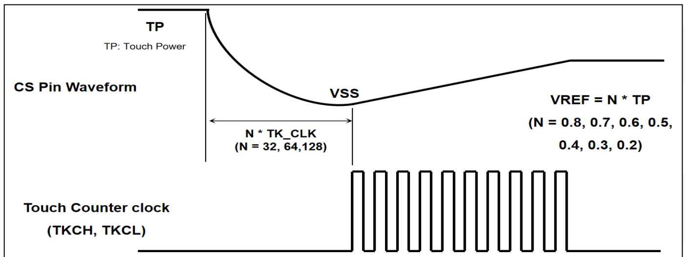
图 42：触摸转换的时序图
