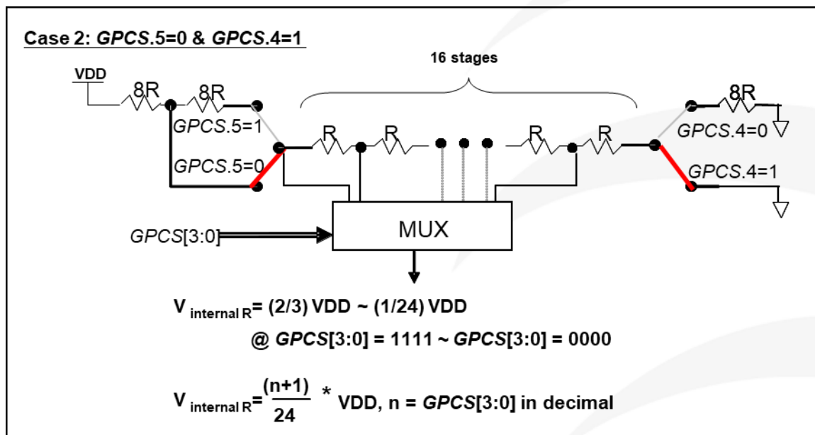
图 32: V_{\text{internal R}} 硬件接法 ( \text{GPCS}.5=0 & \text{GPCS}.4=1 )
