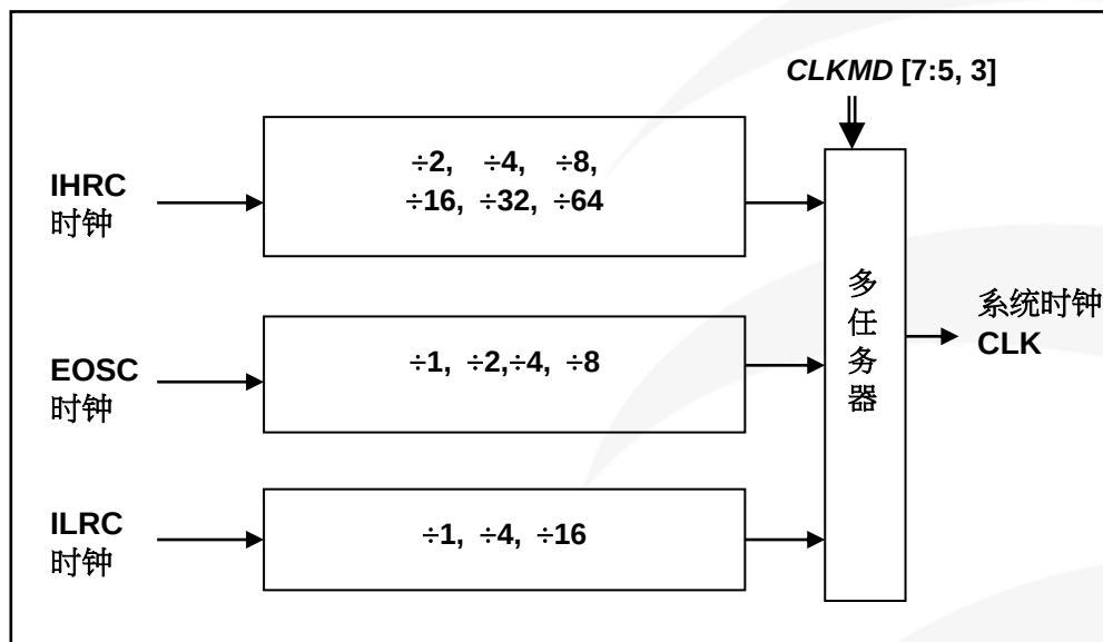
图 2：系统时钟源选择
