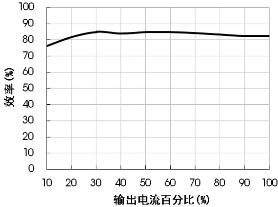
效率Vs输出负载（Vin=5V）
