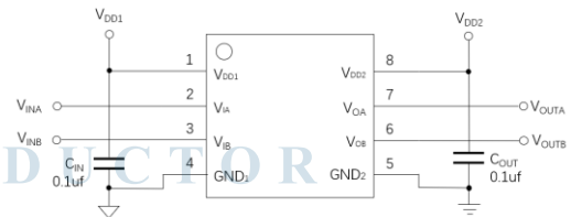
图 3. \pi 120xxx 应用简图
