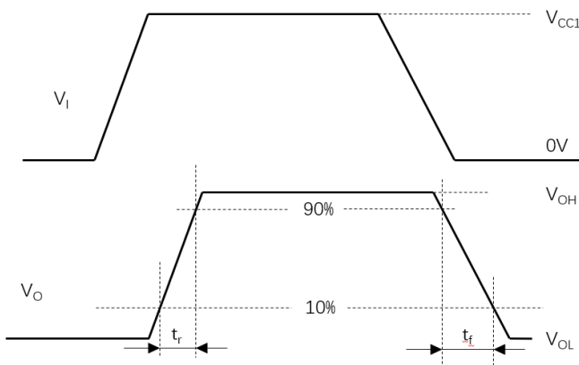
图 8.传输时间波形测量
