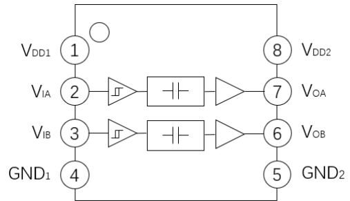
图 1. \pi 120E1x 功能框图
