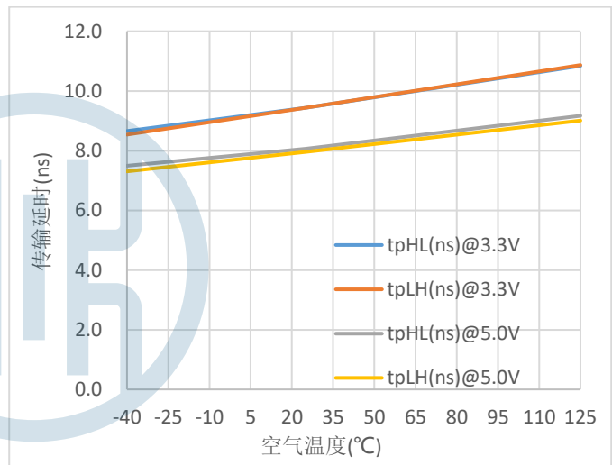
图 7.传输延时 vs. 空气温度
