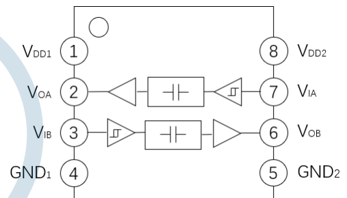
图 2. \pi 122E1x 功能框图
