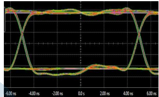
图 11. \pi 12xE1x 眼图
