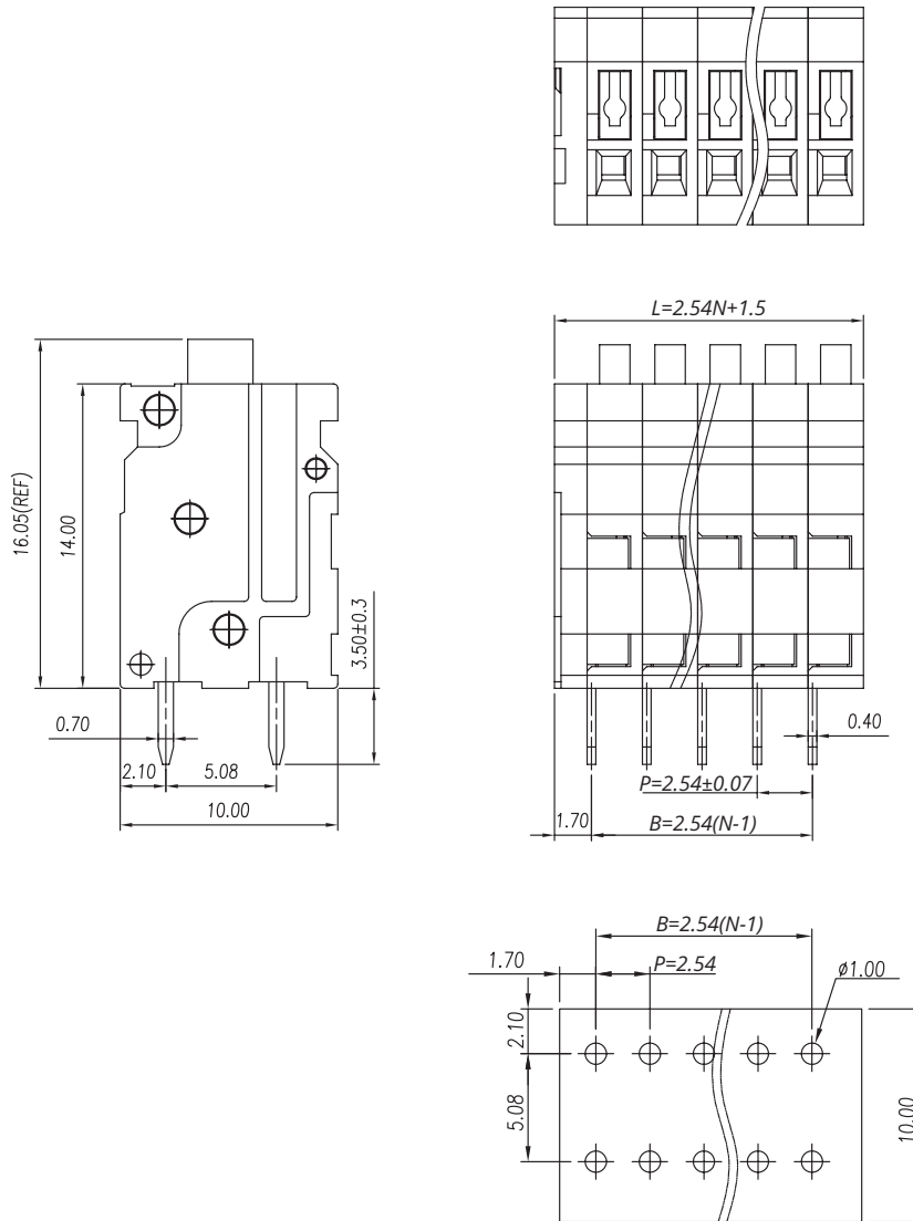
P.C.B. LAYOUT
