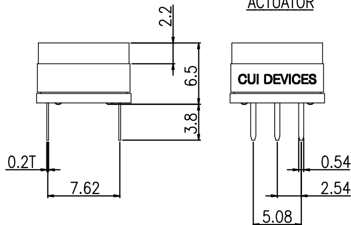
ACTUATOR
