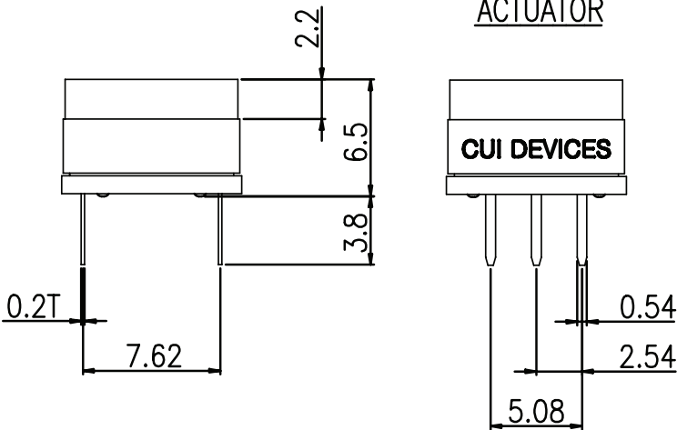
ACTUATOR
