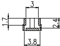
Section A-A' ACTUATOR
