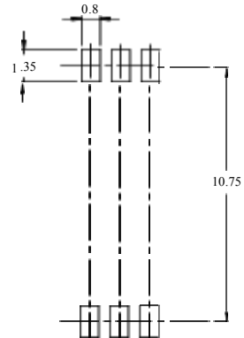
SOP6-W
