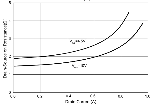
Fig. 4 - R_{DS(ON)} - I_D
