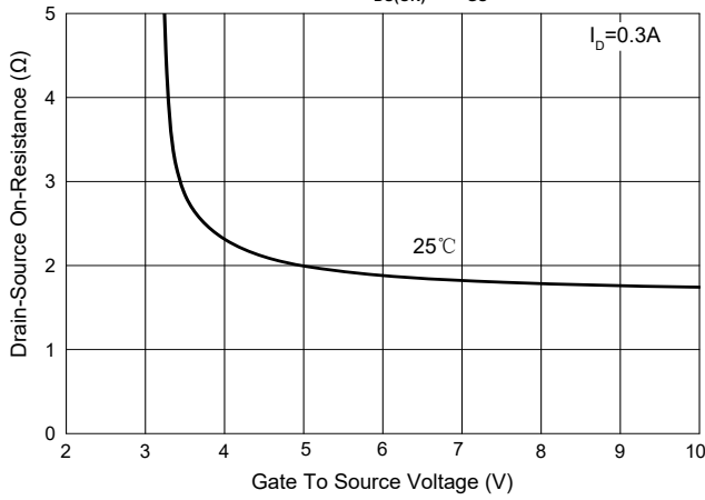
Fig. 3 - R_{DS(ON)} - V_{GS}
