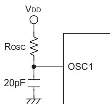
外部 RC 振荡器 – ERC
