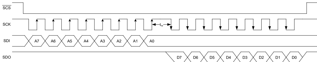
读类型格式：8-bit 命令输入 +8-bit 数据输出
