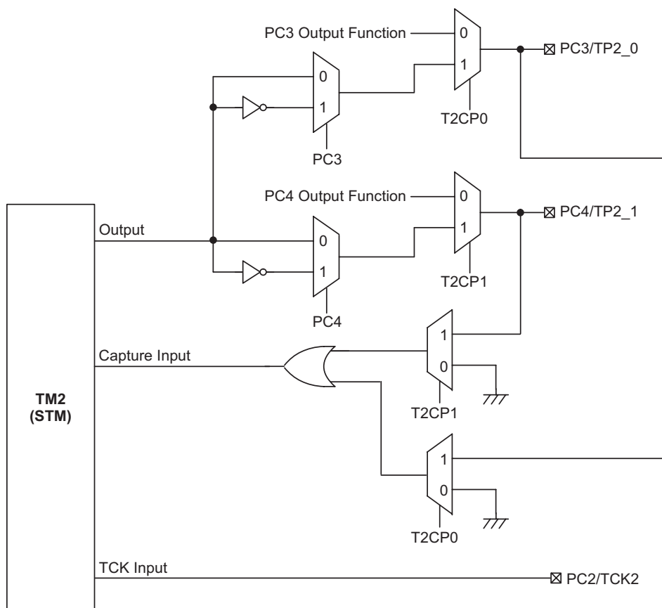
HT66F40 TM0&TM2 功能引脚控制方框图
