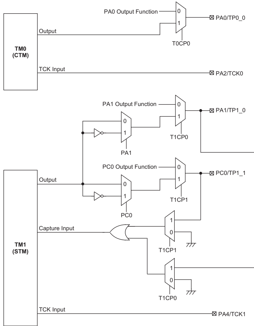
HT66F20 TM 功能引脚控制方框图
