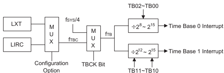
时基中断
