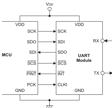
MCU 与 UART 内部连接图
