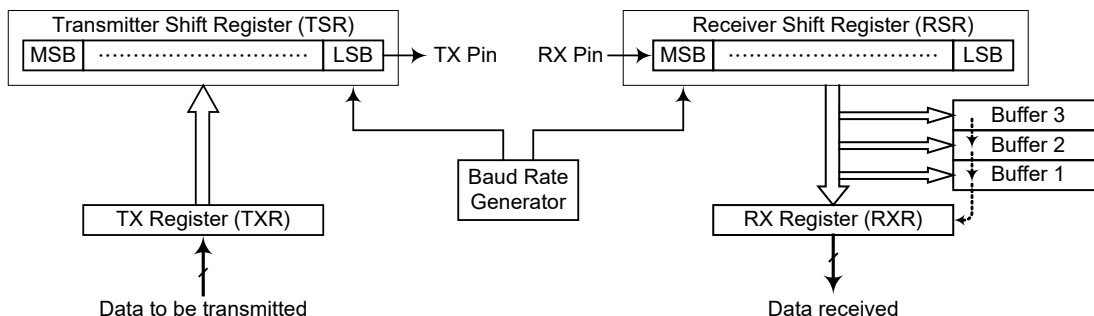
UART 数据传输方案
