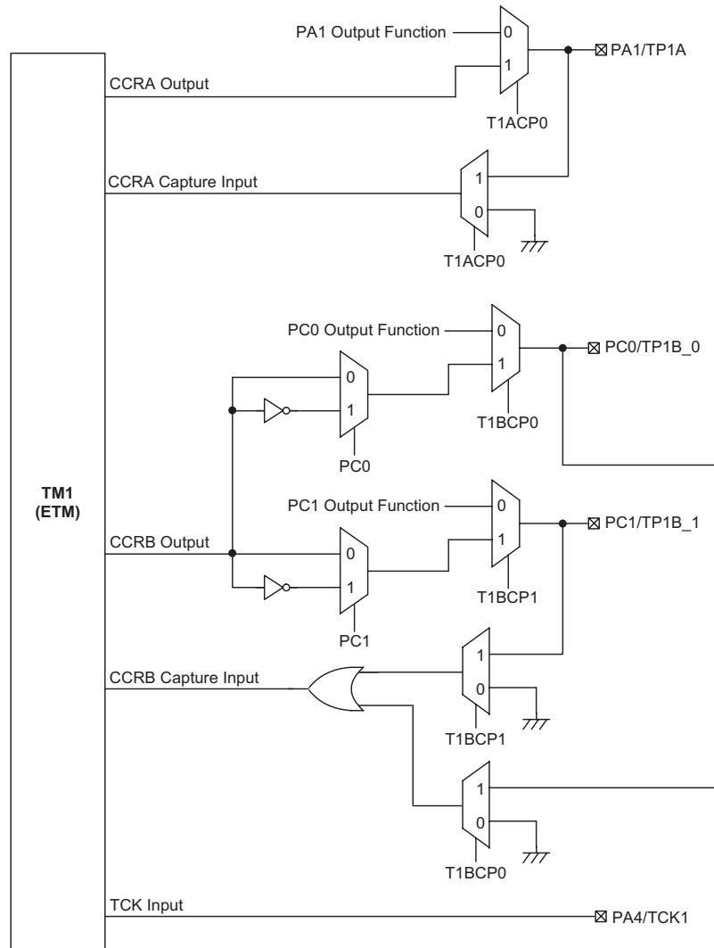
HT66F30 TM 功能引脚控制方框图
