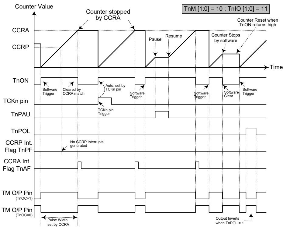
单脉冲模式
