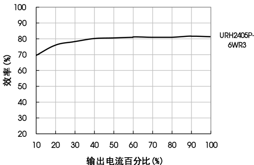
效率Vs输出负载（标称输入）
