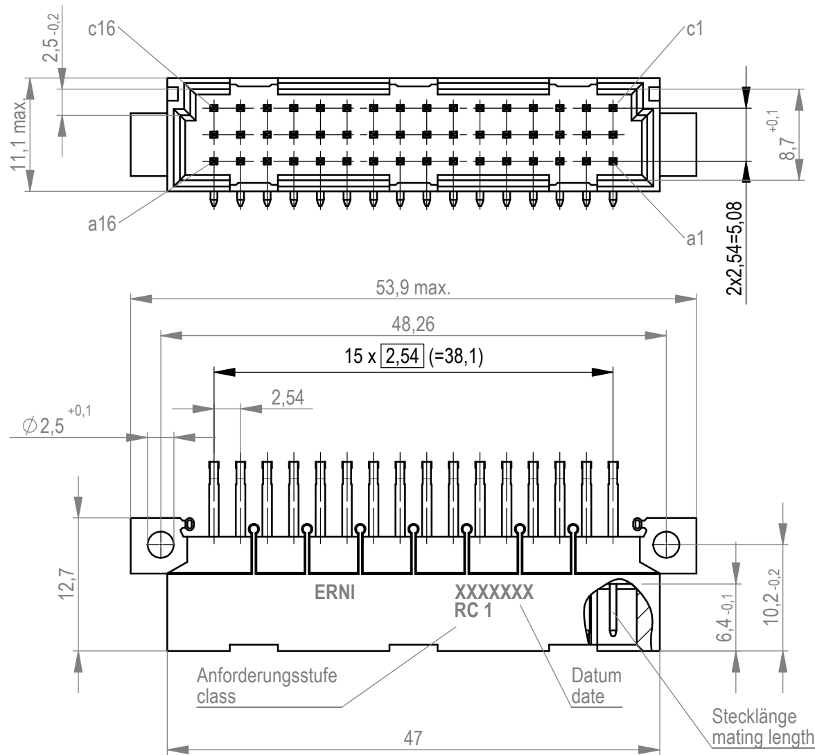
Bestückungsplan / contact layout
