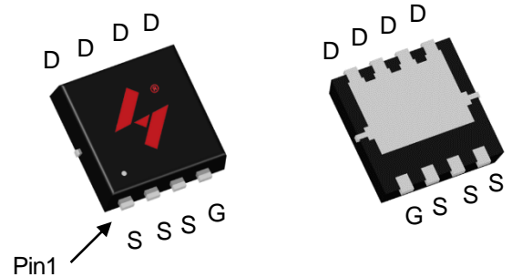
PDFN8L(3.3*3.3)
