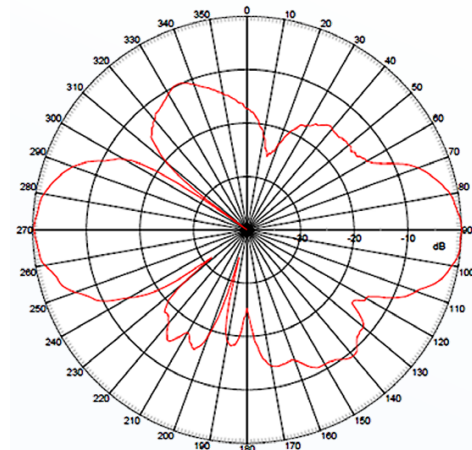
E-plane 5.5 GHz
