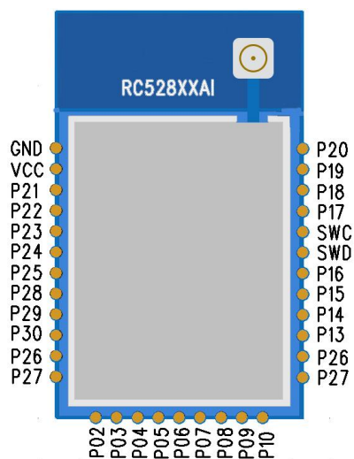
RC52810AI 模块引脚图
