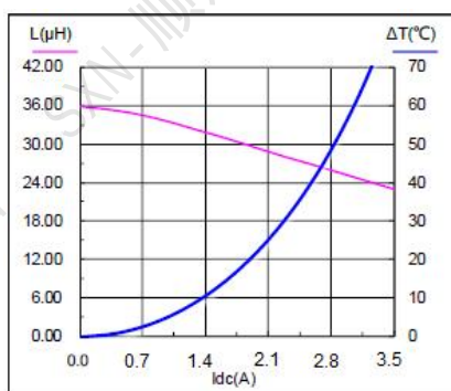
SMMS0630-330M
