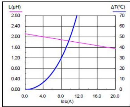
SMMS0630-2R2M
