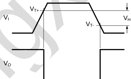
图7 传输特性的定义
