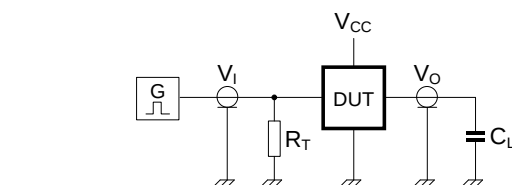
图4 测量开关时间的测试电路
