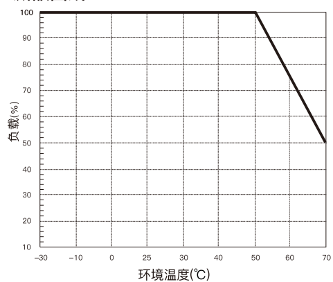
减额曲线
