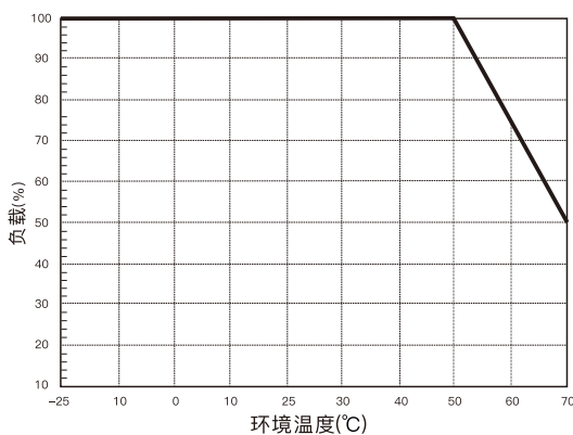
减额曲线
