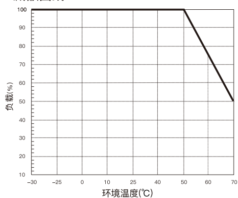
减额曲线
