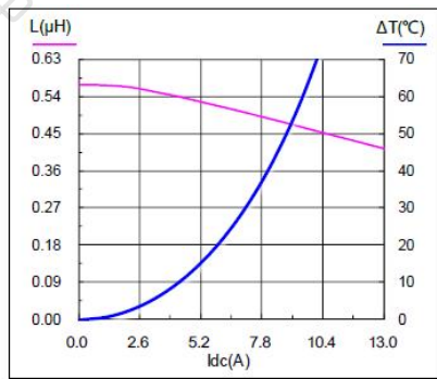
SMS0420-R56M
