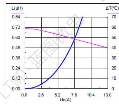
SMS0420-R68M
