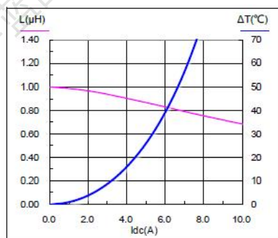
SMS0420-1R0M
