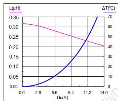
SMS0420-R68M
