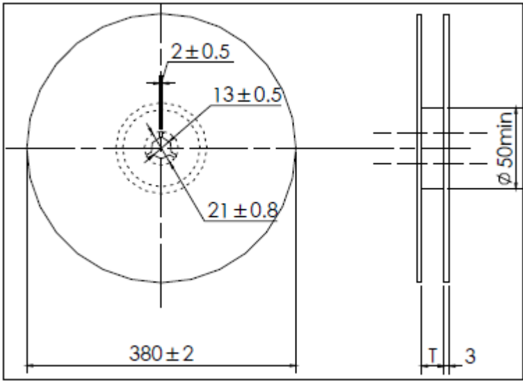
编带包装盘 Reel
