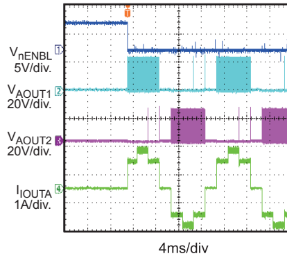
Enable-Half Step
