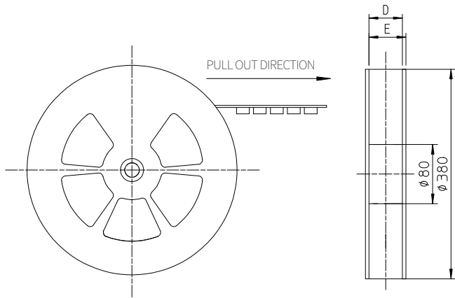
Reel Dimensions
