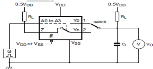
a. Test circuit
