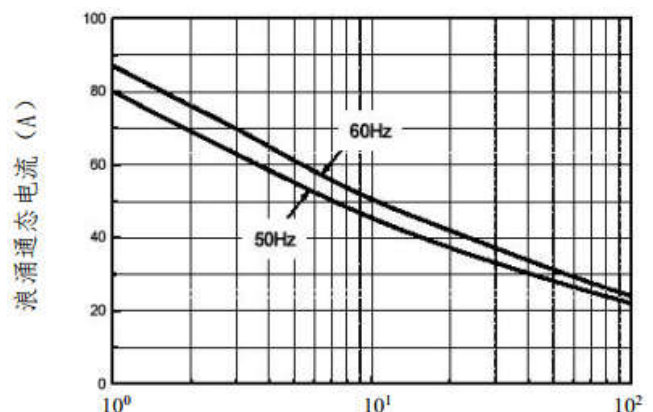
时间 (Cycles)
