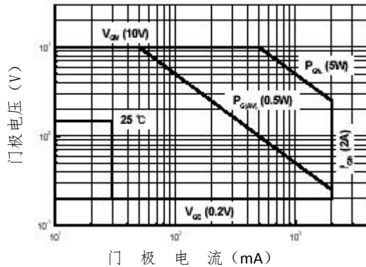
图一、门极特性
