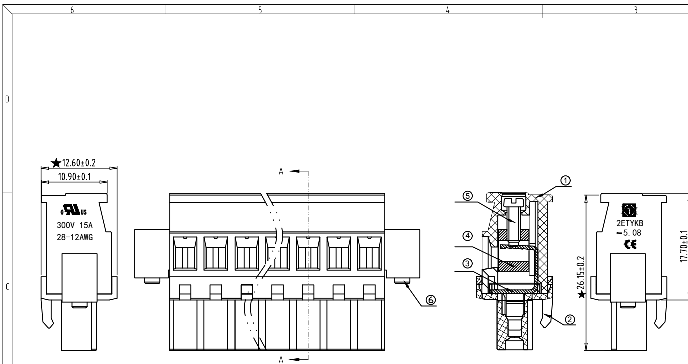
SECTION A-A
