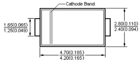
SMA (DO-214AC)
