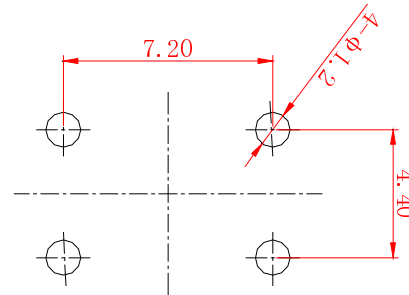
PCB 参考图
