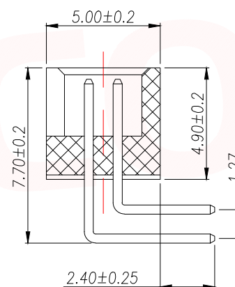
A-A SECTION
