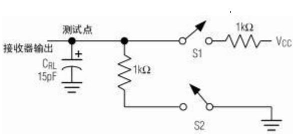
图1：接收器时序测试电路
