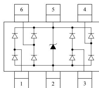
SOT23-6L
