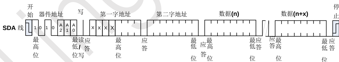
图 9、页写
