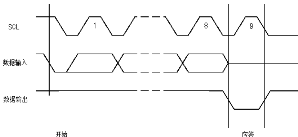
图 7、输出响应
