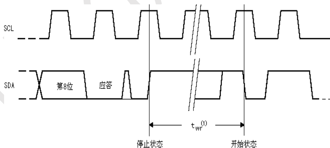
图 6、写周期时序
