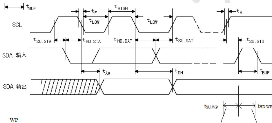
图 5、总线时序
