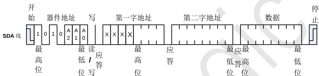
图 8、字节写
