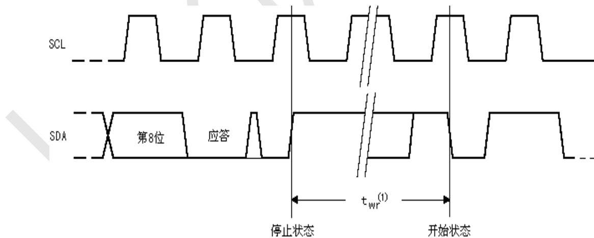
图 6、写周期时序
