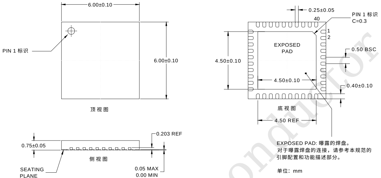
图 15: 封装信息
