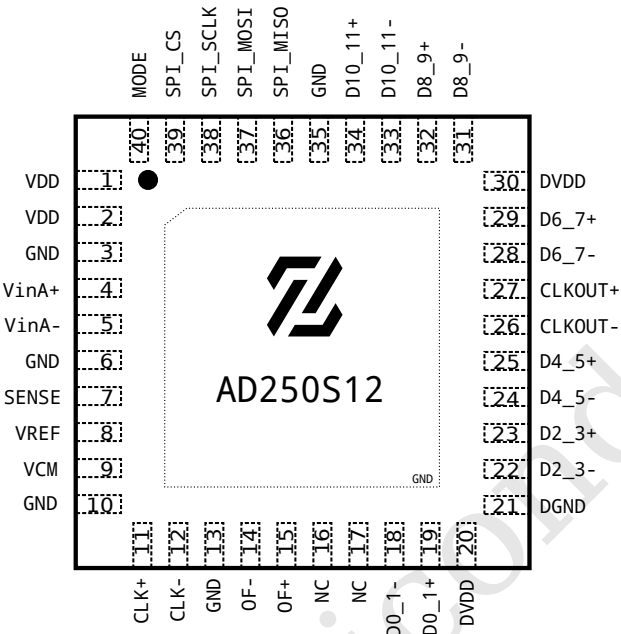
图 4: 正面视图 6mmx6mmQFN40 封装
