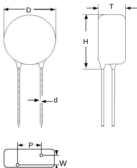
两脚N型
