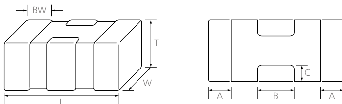
Low ESL Capacitor_3T
