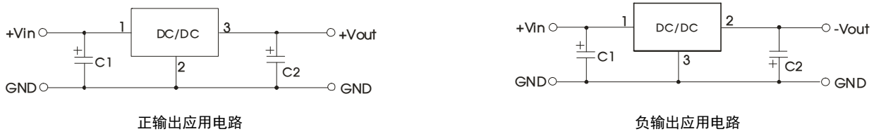
图 2 典型应用电路
