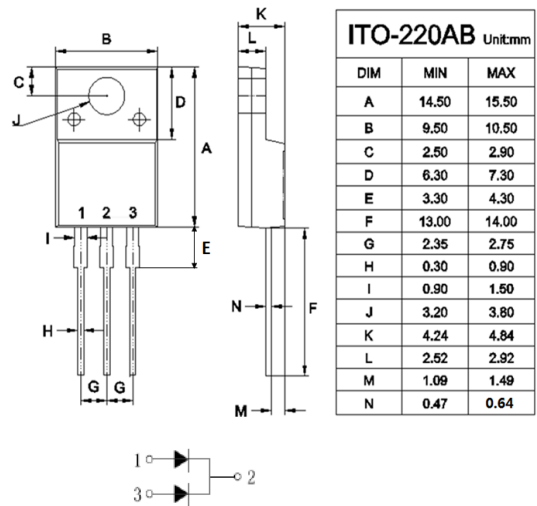
ITO-220AB
