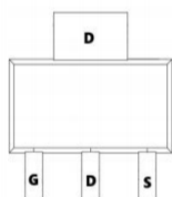
SOT89-3
