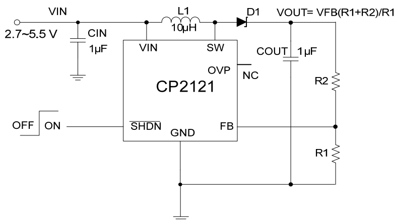
图 2 CP2121 应用图 1
