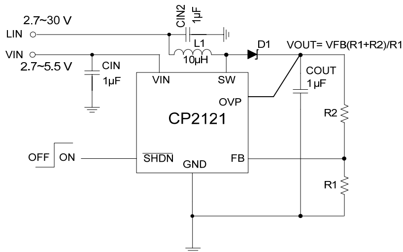
图 3 CP2121 应用图
