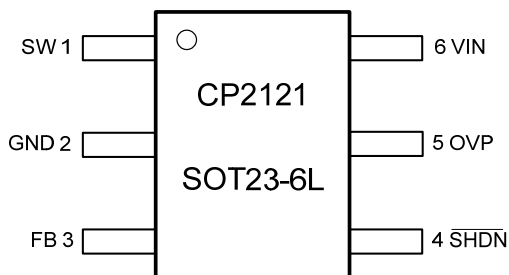
图 1 CP2121 封装引脚图
