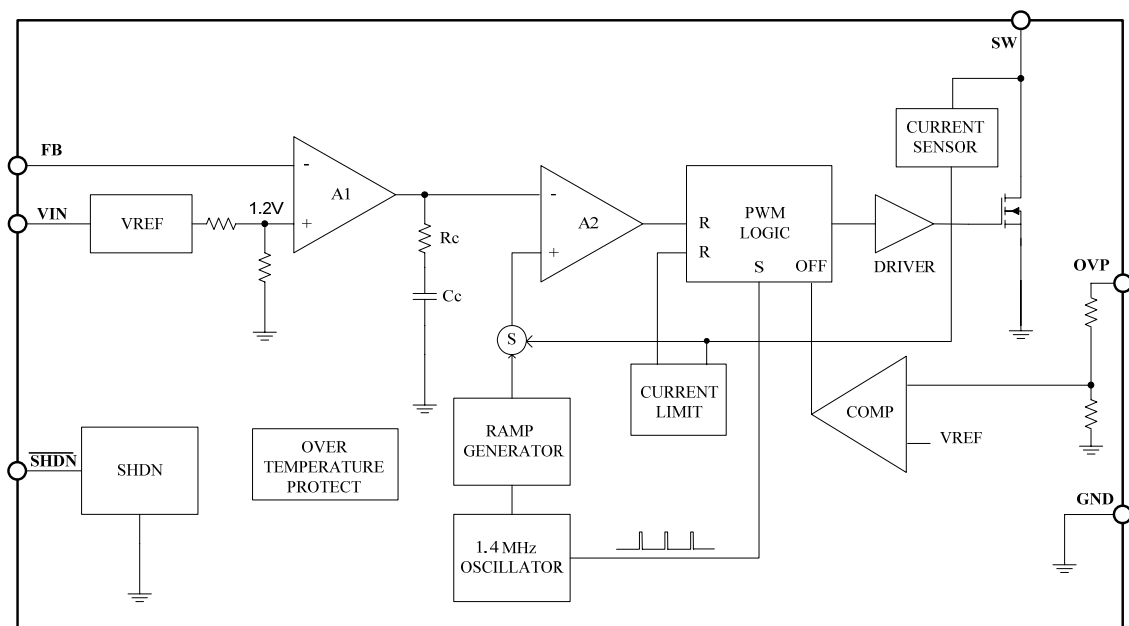
图 4 CP2121 功能方框图
