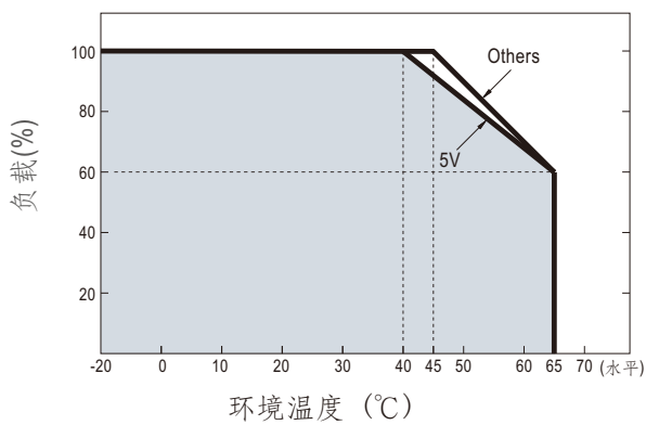
■ 减额曲线
