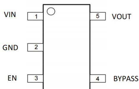
SOT23-5
