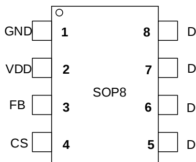
图 2 管脚封装图
