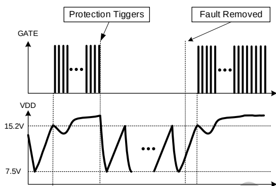
图 5 保护波形图
