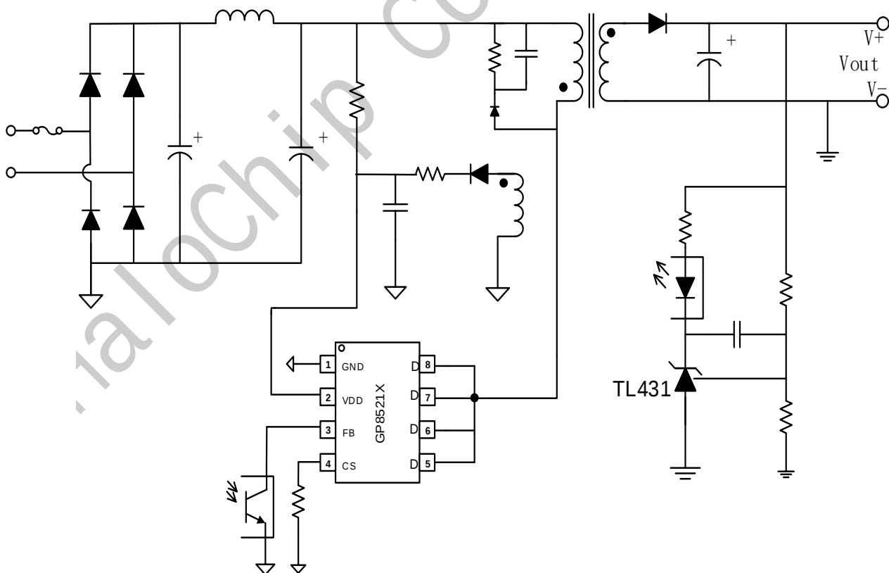
图 1 GP8521X 典型应用图
