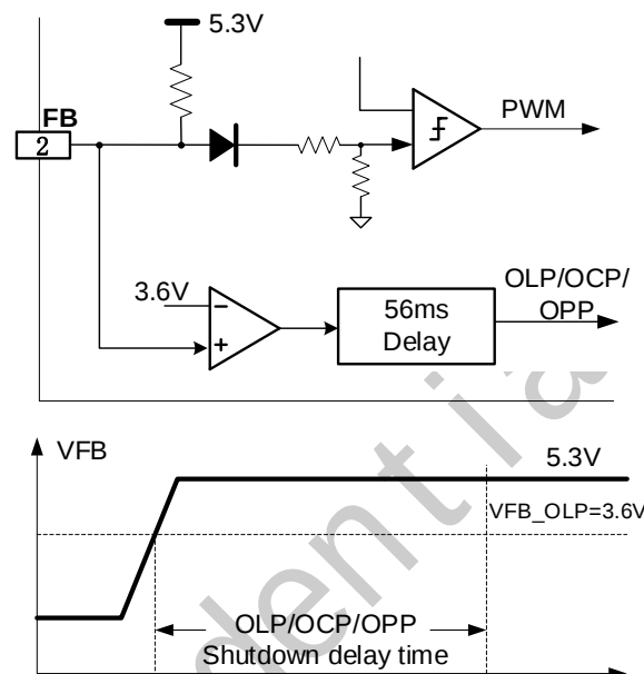
图 6 保护延时波形
