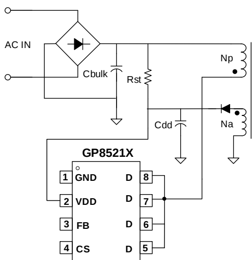
图 3 典型的启动电路
