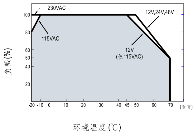
■ 减额曲线
