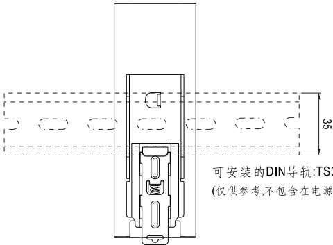
背面图
