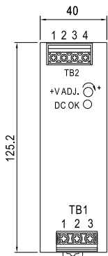
前视图
