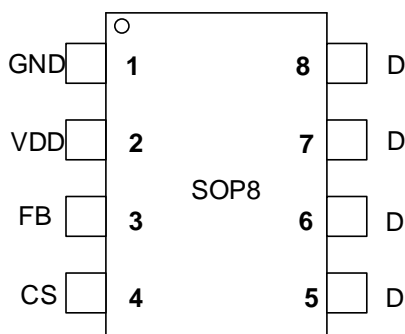
图 2 管脚封装图
